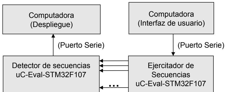
Figura 7. Diagrama a bloques de la aplicación
