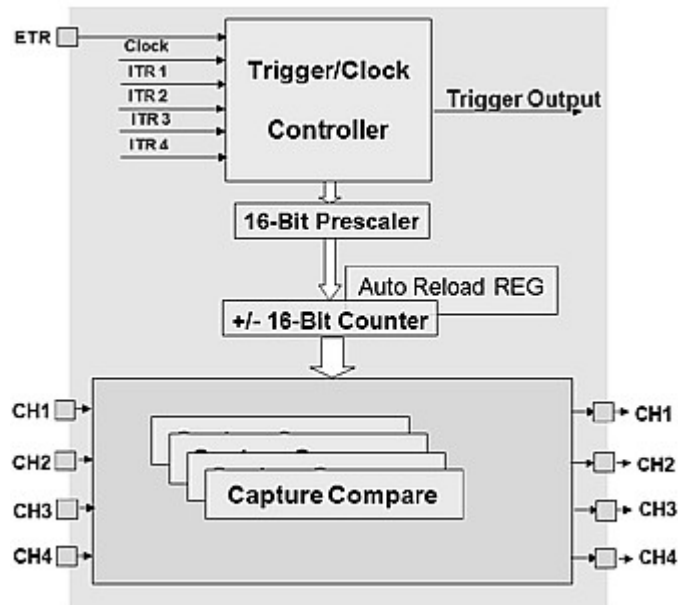
Figura 10. Timer genérico de la familia STM32
