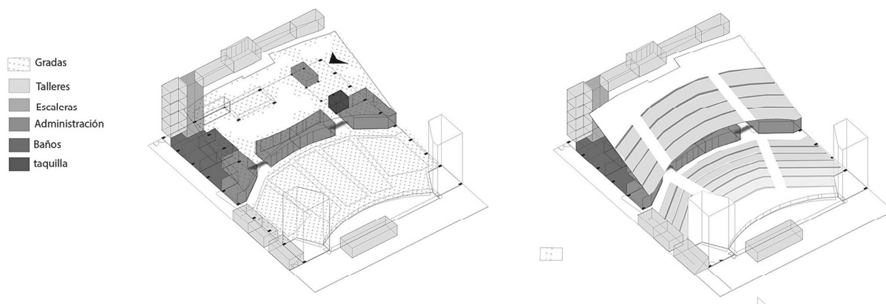
Isométricos del Centro de Arte y Cultura Circo Volador vista desde el sureste.
