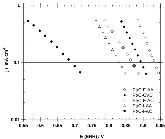
Figura 3.17 Pendientes de Tafel para compuestos de Pt/C sintetizados por impregnación, foto-depósito y CVD utilizando \text{H}_2\text{PtCl}_6 y \text{C}_{10}\text{H}_{14}\text{O}_4\text{Pt} como precursores.
