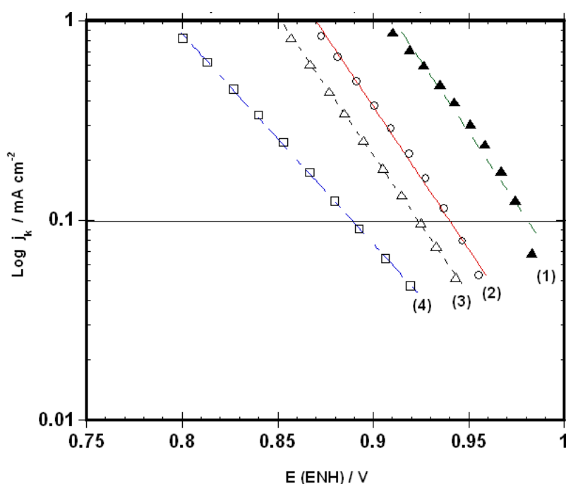
Figura 4.20 Gráfico de Tafel de los catalizadores sintetizados por foto-depósito (1)10%Pt-5%TiO 2 -C-259-B y (3)10%Pt-15%TiO 2 -112-B. Por CVD (2)10%Pt-5%TiO 2 -C-CVD y (4) 10%Pt-15%TiO 2 -C-CVD.
