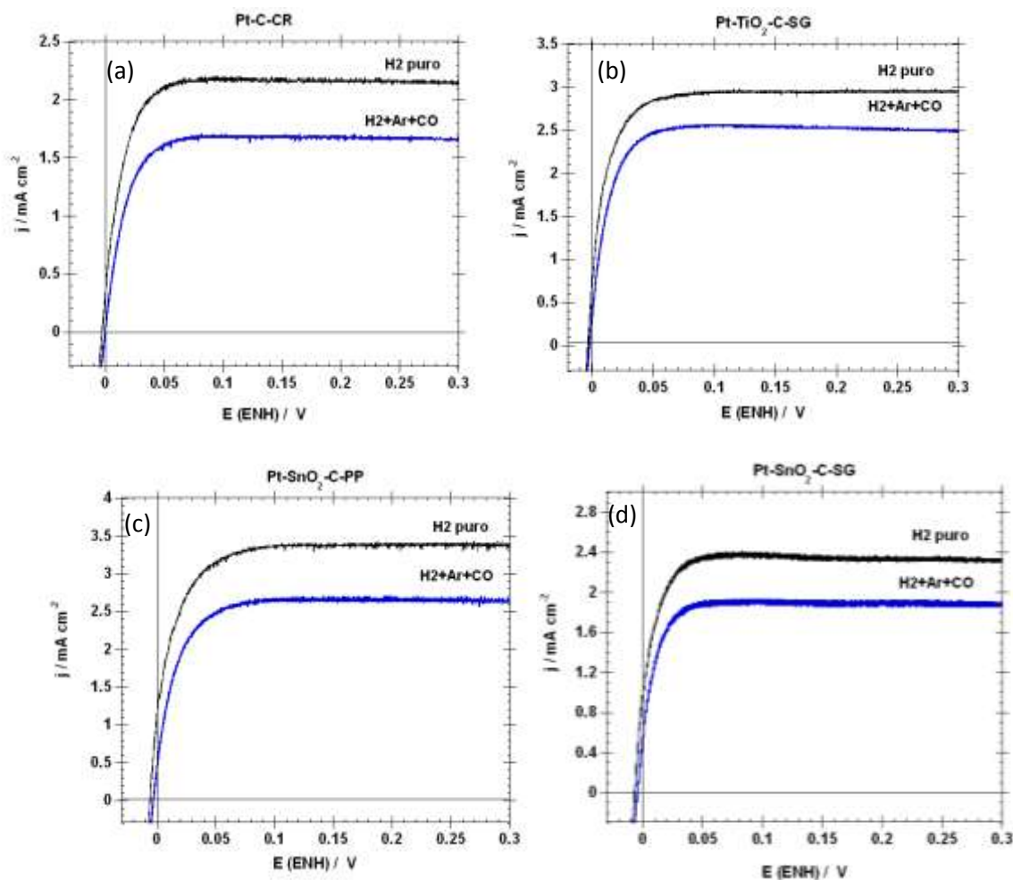
Figura 6.11 Curvas de corriente-potencial para la oxidación de hidrógeno ( H_2 ) y una mezcla gaseosa de H_2+Ar con 100 ppm de CO a 2000 rpm en H_2SO_4 0.5 M a 25 °C a 1mVs^{-1} sobre los catalizadores (a) Pt-C, (b) Pt-TiO 2 -C-SG, (c) Pt-SnO 2 -C-PP y (d) Pt-SnO 2 -C-SG.
