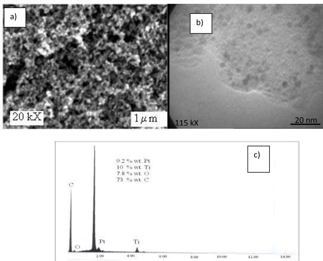
Figura 4.3 a) Imagen de SEM, b) imagen de TEM y c) análisis EDS del catalizador 10%Pt/15% \text{TiO}_2 /C-20-B.
