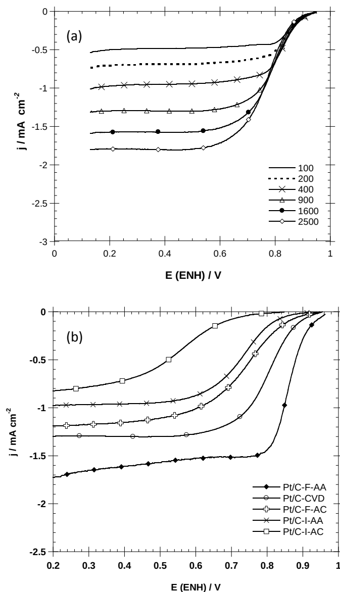
Figura 3.16 a) Voltametría lineal del catalizador 10%Pt/C-CVD preparados con \text{C}_{10}\text{H}_{14}\text{O}_4\text{Pt} . b) RRO a 900 rpm sobre los diferentes catalizadores preparados de 10%Pt/C. En \text{H}_2\text{SO}_4 0.5 M a 25^\circ\text{C} y 5\text{mVs}^{-1} .
