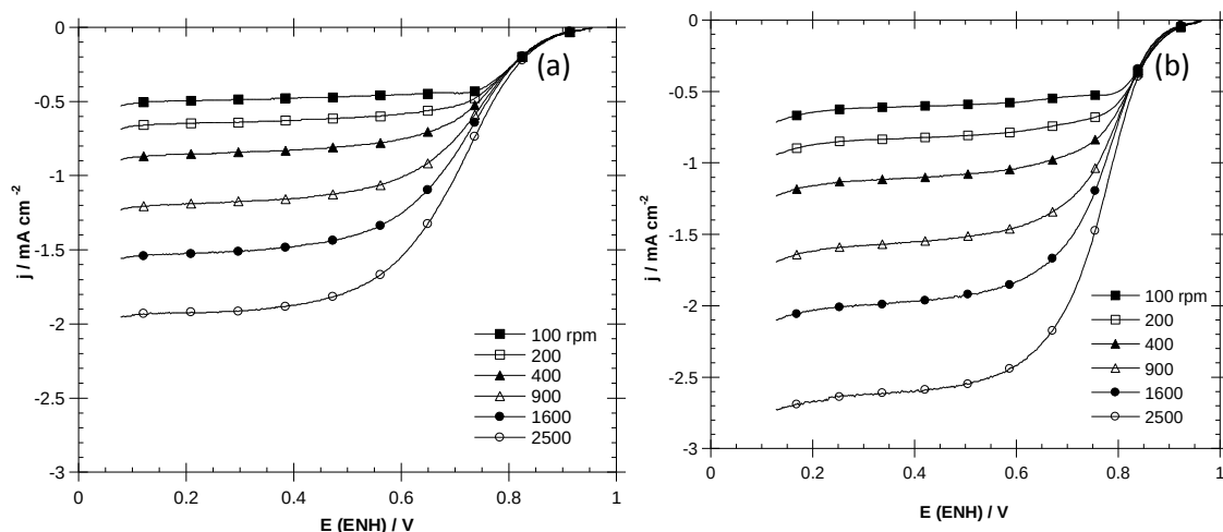
Figura 3.14 Voltametría lineal de los compuestos sintetizados por foto-depósito químico: a) 10%Pt/C-F-AC, b) 10%Pt/C-F-AA, preparados con \text{H}_2\text{Cl}_6\text{Pt} y \text{C}_{10}\text{H}_{14}\text{O}_4\text{Pt} . En \text{H}_2\text{SO}_4 0.5 M a 5 \text{ mV s}^{-1} .
