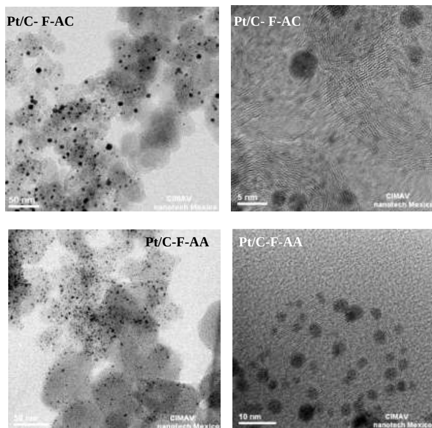
Figura 3.9 Imágenes de TEM de los catalizadores 10%Pt/C-F-AC y 10%Pt/C-F-AA sintetizados por el método de fotodepósito \text{H}_2\text{PtCl}_6 y \text{C}_{10}\text{H}_{14}\text{O}_4\text{Pt} como precursores.
