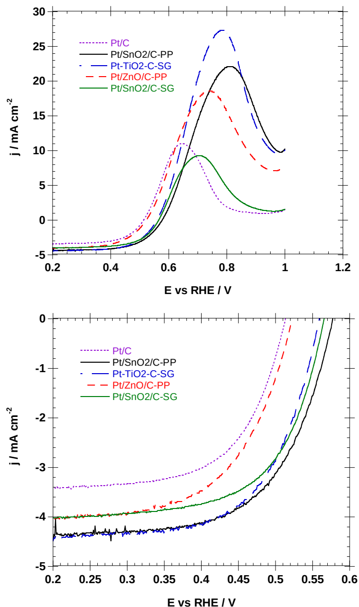
Figura 6.10 Comparación de las curvas de polarización de la RRO en presencia de metanol a 900 rpm, sobre los catalizadores 8%Pt-C-CR, 10%Pt5%TiO 2 -C-SG, 10%Pt5%SnO 2 -C-SG, 10%Pt5%SnO 2 -C-PP y 10%Pt5%ZnO-C-PP. Electrolito de H 2 SO 4 0.5 M + CH 3 OH 0.5 M 5 mV s -1 y 25°C.
