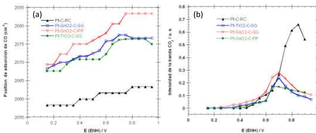
Figura 5.5 (a) Posición de la banda de CO y (b) Integración de la intensidad de la banda generada de \text{CO}_2 en función del potencial aplicado sobre los catalizadores 10%Pt/C y 10%Pt/5%óxido/C preparados por foto-depósito químico.
