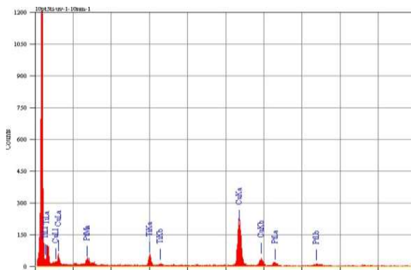
Figura 4.6 Imágenes de TEM y EDS del catalizador 10%Pt/5%TiO 2 /C-259-B sintetizado mediante foto-catálisis con la lámpara de 259W y 5% TiO 2 .
