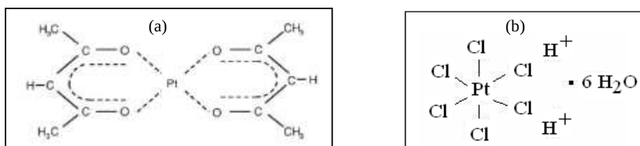
Figura 2.2 Representación esquemática de los precursores de Pt utilizados (a) acetyl-acetonato de Pt, AA ( \text{C}_{10}\text{H}_{14}\text{O}_4\text{Pt} ) y (b) ácido hexacloroplatínico, AC ( \text{H}_2\text{PtCl}_6 ).
