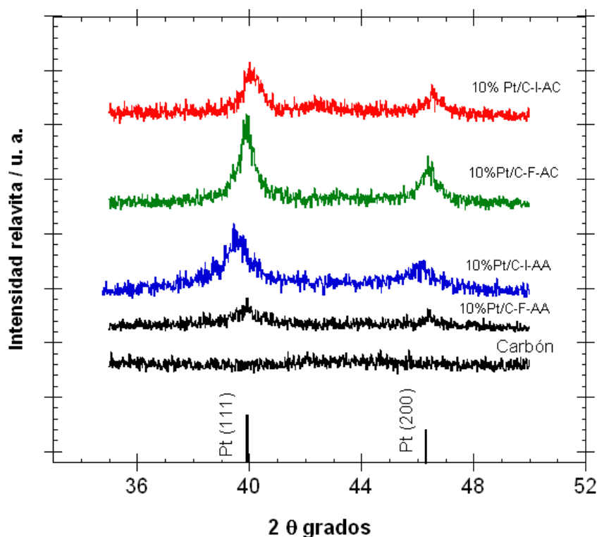
Figura 3.6 Patrones de Difracción de Rayos X de catalizadores de 10%Pt/C preparados por impregnación y fotodeposición.
