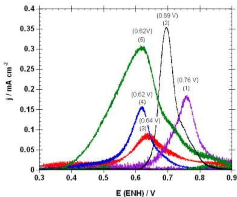
Figura 5.8 Oxidación de CO sobre los electrocatalizadores (1) 8%Pt/C, (2) 10%Pt-5%TiO 2 -C-SG, (3) 10%Pt-5%ZnO-C, (4) 10%Pt-5%SnO 2 -C-SG en y (5) 10%Pt-5%SnO 2 -C-PP H 2 SO 4 0.5 M saturado de CO a una velocidad de 5 \text{ mVs}^{-1} y 25^\circ\text{C} . 0.420 \text{ mC cm}^{-2} corresponde a una monocapa de CO adsorbida [8] .
