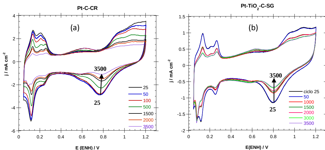
Figura 6.1. Estabilidad electroquímica del catalizador (a) 10%Pt-C-CR y (b) 10%Pt-5%TiO 2 -C-SG durante 3500 ciclos de voltametría cíclica en \text{H}_2\text{SO}_4 0.5 M, atmosfera de \text{N}_2 a una velocidad de 50 \text{ mV s}^{-1} . T = 25^\circ\text{C} .
