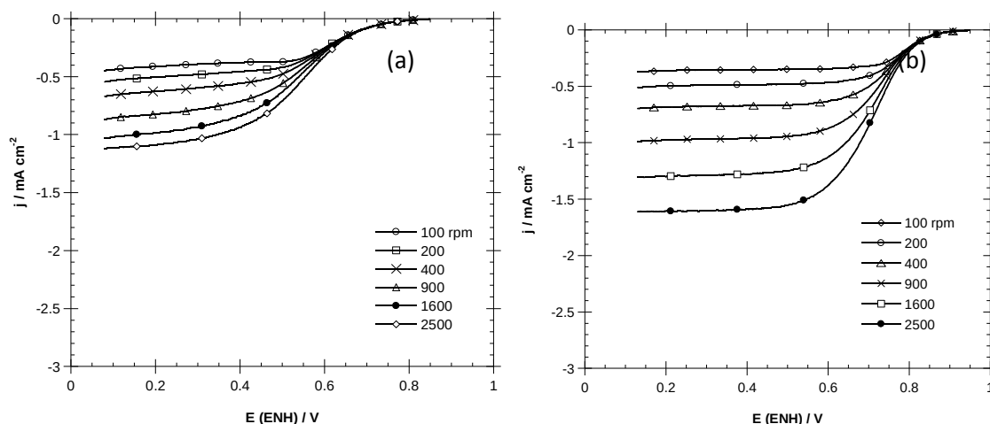
Figura 3.15 Voltametría lineal de los compuestos sintetizados por el método de impregnación: a) 10%Pt/C-I-AC, b) 10%Pt/C-I-AA, preparados con \text{H}_2\text{Cl}_6\text{Pt} y \text{C}_{10}\text{H}_{14}\text{O}_4\text{Pt} . En \text{H}_2\text{SO}_4 0.5 M a 5 \text{ mV s}^{-1} .
