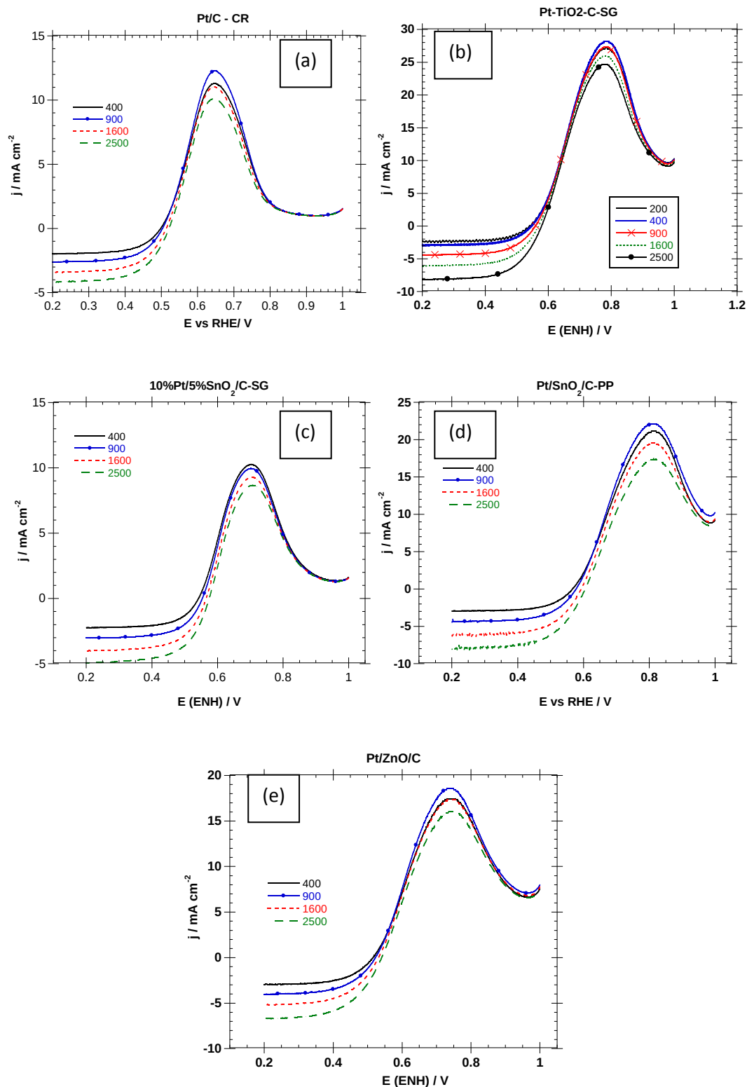
Figura 6.9 Reacción de reducción de oxígeno en presencia de metanol (a) 8%Pt-C-CR, (b) 10%Pt5%TiO 2 -C-SG, (c) 10%Pt5%SnO 2 -C-SG, (d) 10%Pt5%SnO 2 -C-PP y (e) 10%Pt5%ZnO-C-PP a diferentes velocidades de rotación (400, 900, 1600 y 2500 rpm). Electrolito de H 2 SO 4 0.5 M + CH 3 OH 0.5 M 5 mV s -1 y 25°C.
