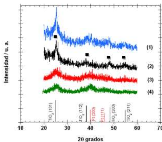
Figura 4.1 Patrones de difracción de rayos-X de los catalizadores (1)10%Pt-15% \text{TiO}_2 -C-112-A, (2)10%Pt- \text{TiO}_2 -112-A, (3)10%Pt-15% \text{TiO}_2 -C-112-B y (4) 10%Pt-5% \text{TiO}_2 -20-B.
