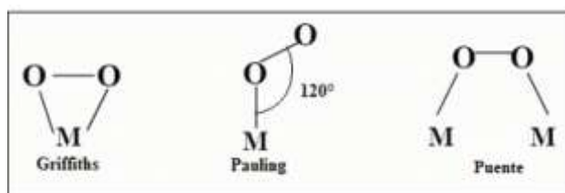
Figura 1.6. Modelos propuestos por Yeager para la interacción entre el oxígeno y el electrocatalizador.
