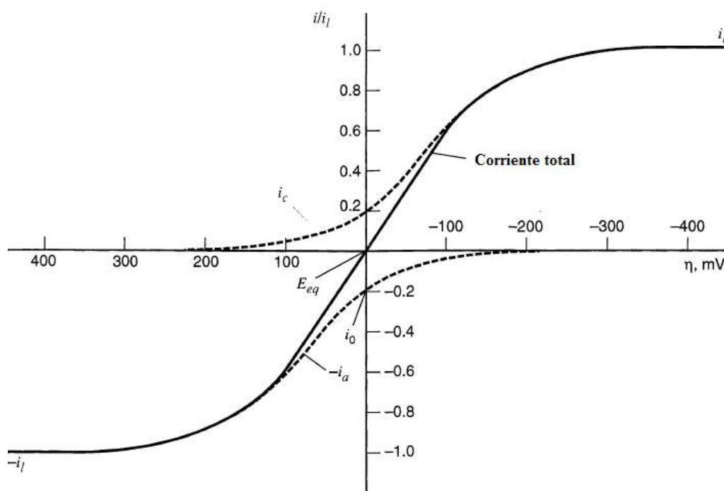
Figura 1.7 Curvas de corriente-sobrepotencial para el sistema O + e^- \rightarrow R , con \alpha=0.5 , T = 298 \text{ K} , i_{l,c} = i_{l,a} = i_l y i_o = 0.2 . Las líneas punteadas corresponden a la corriente catódica y anódica [14] .
