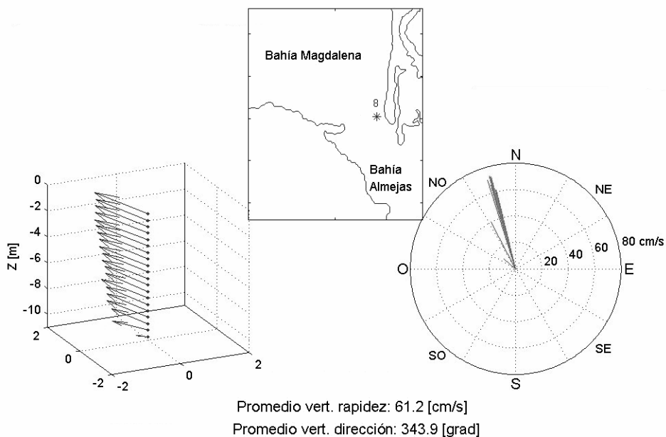
Figura 34. Perfil de la corriente obtenido con un ADCP en el Canal Gaviotas en Abril del 2000 durante el reflujó de marea.
