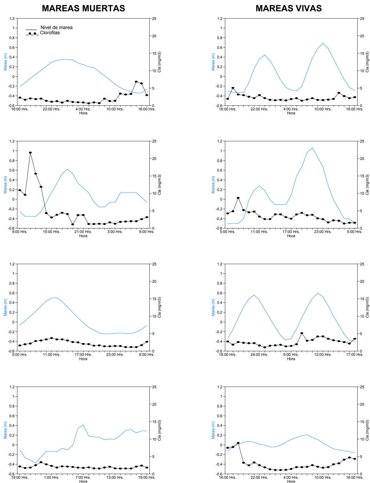
Fig. 17 Variación de las clorofilas el año 2002 en el manglar El Conchalito, para los cuatro muestreos del año (febrero en la primera fila, junio en la segunda, septiembre en la tercera y noviembre en la cuarta fila).
