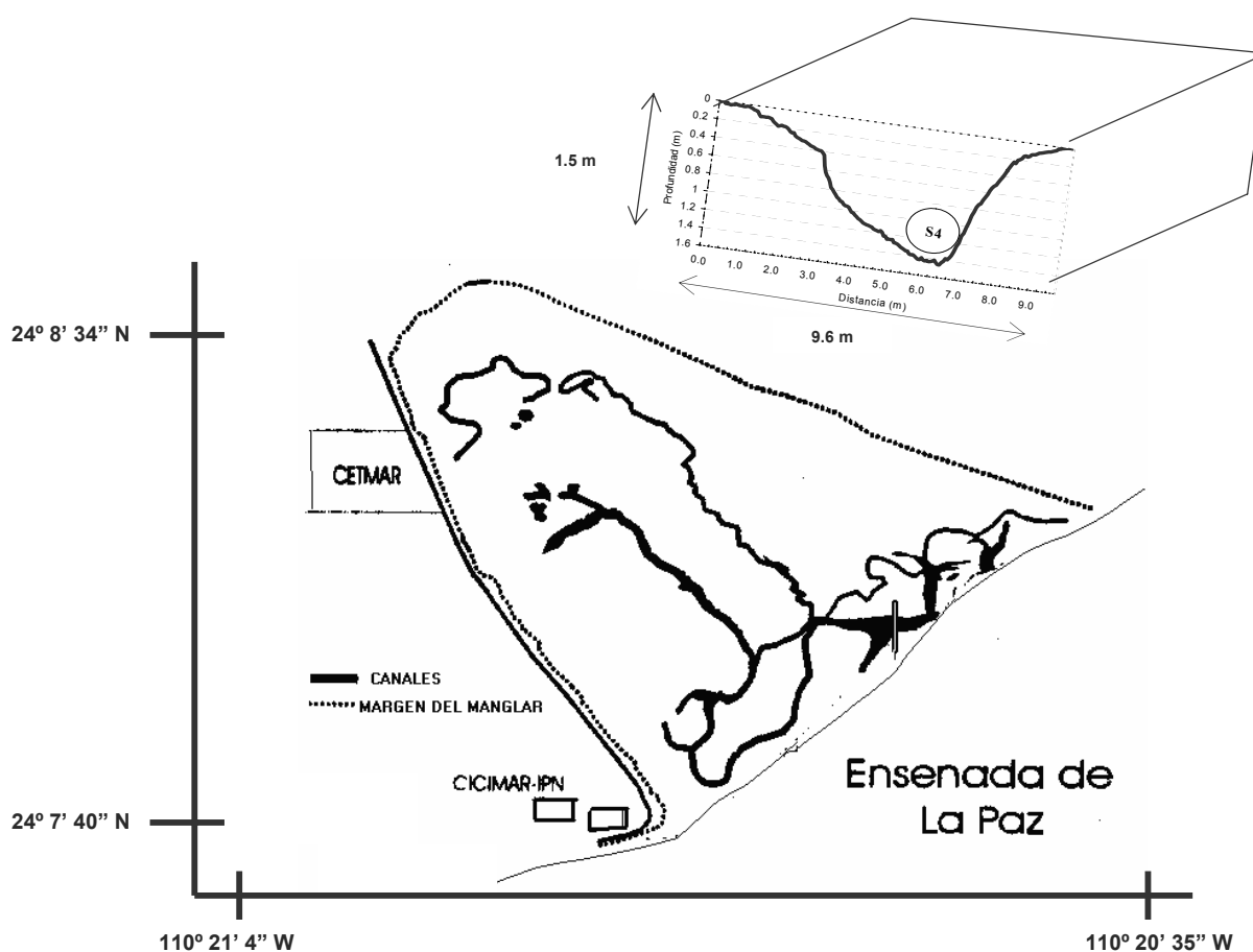
Fig. 2. Detalle del sistema de canales del área de estudio. Se detalla en la sección transversal del canal de mareas en el punto de muestreo, la batimetría del canal y su profundidad máxima, así como el sitio donde se colocó el correntómetro.
