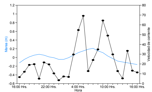
Fig. 3 Relación del nivel de mareas y la velocidad de corriente durante el año 2002 en el manglar El Conchalito, para los cuatro muestreos del año (febrero en la primera fila, junio en la segunda, septiembre en la tercera y noviembre en la cuarta fila).
