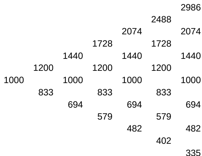
Árbol binomial de 6 periodos
