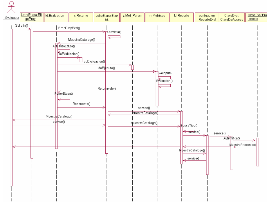
Figura AP.A.7 Diagrama de bajo nivel de la Evaluación individual.
