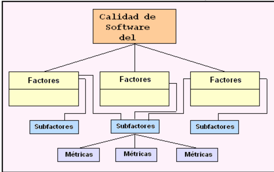
Figura 2.3 Estructura de las métricas de Calidad de Software según el estándar IEEE-1061 [19]
