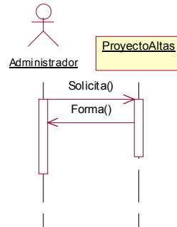
Figura AP.A.4 Diagrama de secuencia de bajo nivel del Registro de Proyectos.
