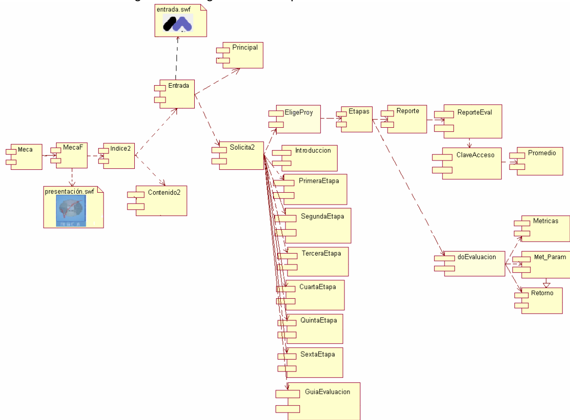
Figura 4.5 Diagrama de componentes del Evaluador Informal .
