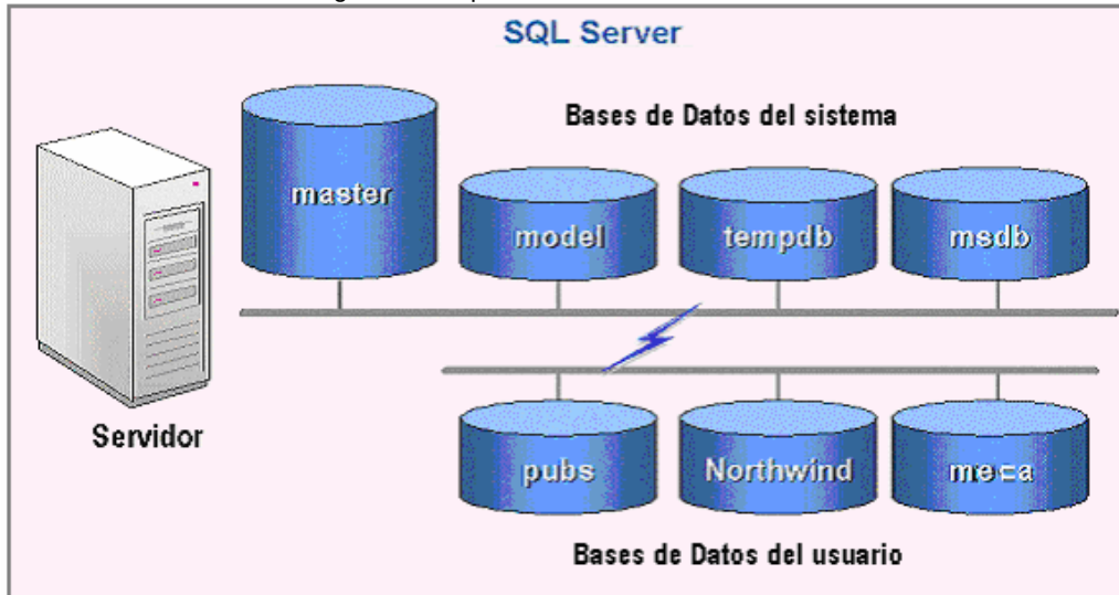
Figura 3.7 Arquitectura de la Base de Datos
