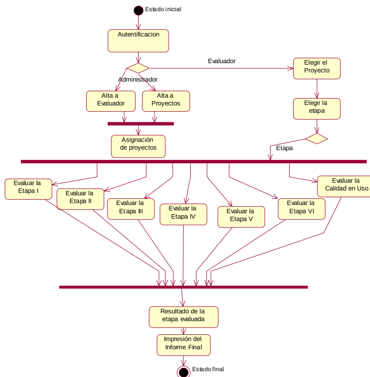
Figura 3.5 Diagrama de actividades del Sistema MECA
