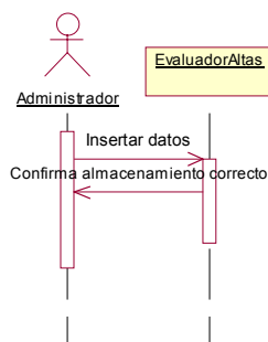
Figura AP.A.1 Diagrama de secuencia de alto nivel de abstracción del Registro de evaluadores.
