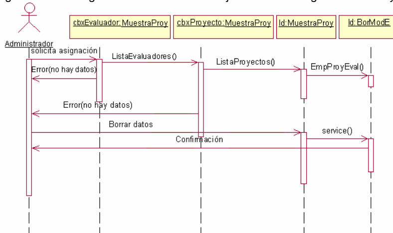
Figura AP.A.6 Diagrama de secuencia de bajo nivel de la Asignación de Proyectos.
