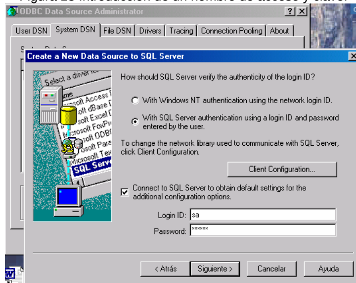
Figura 13 Introducción de un nombre de acceso y clave.
