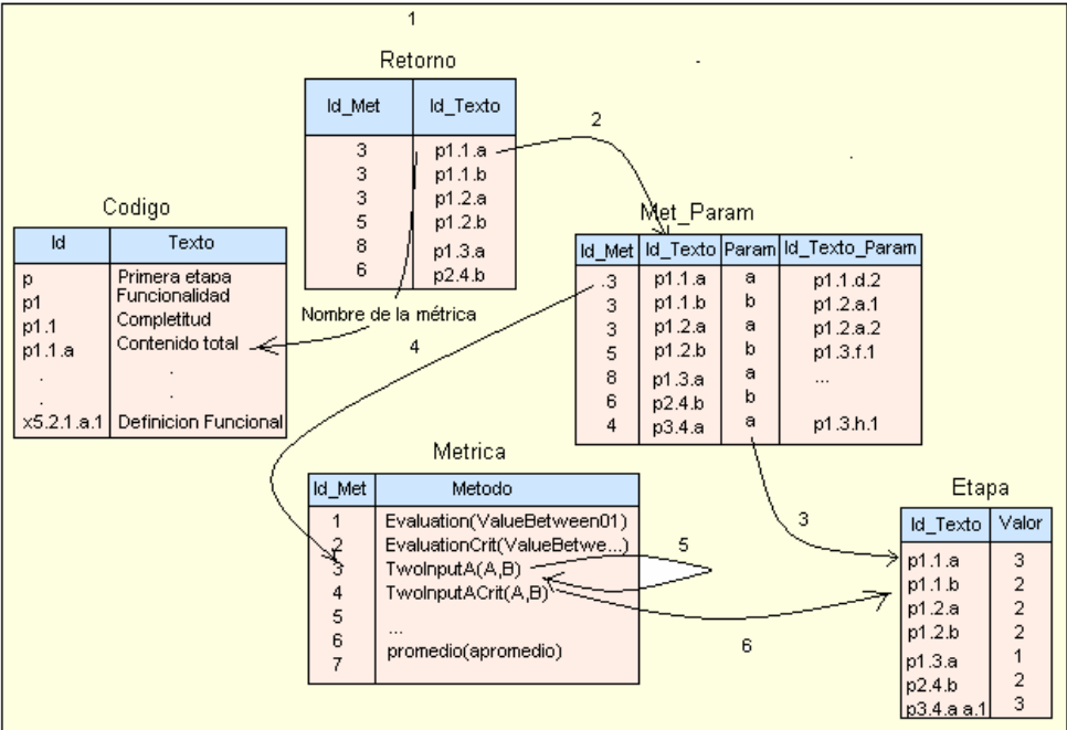
Figura 3.9 Secuencia de ejecución de la Evaluación
