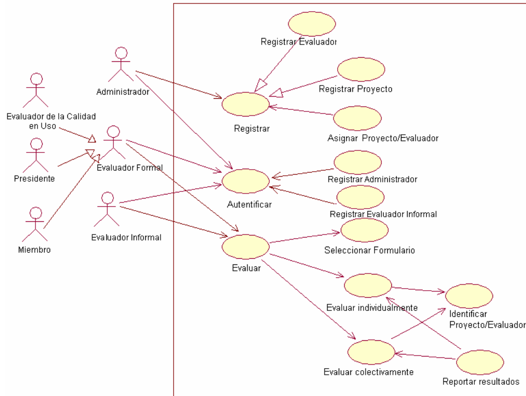
Figura 3.1 Caso de Uso general
