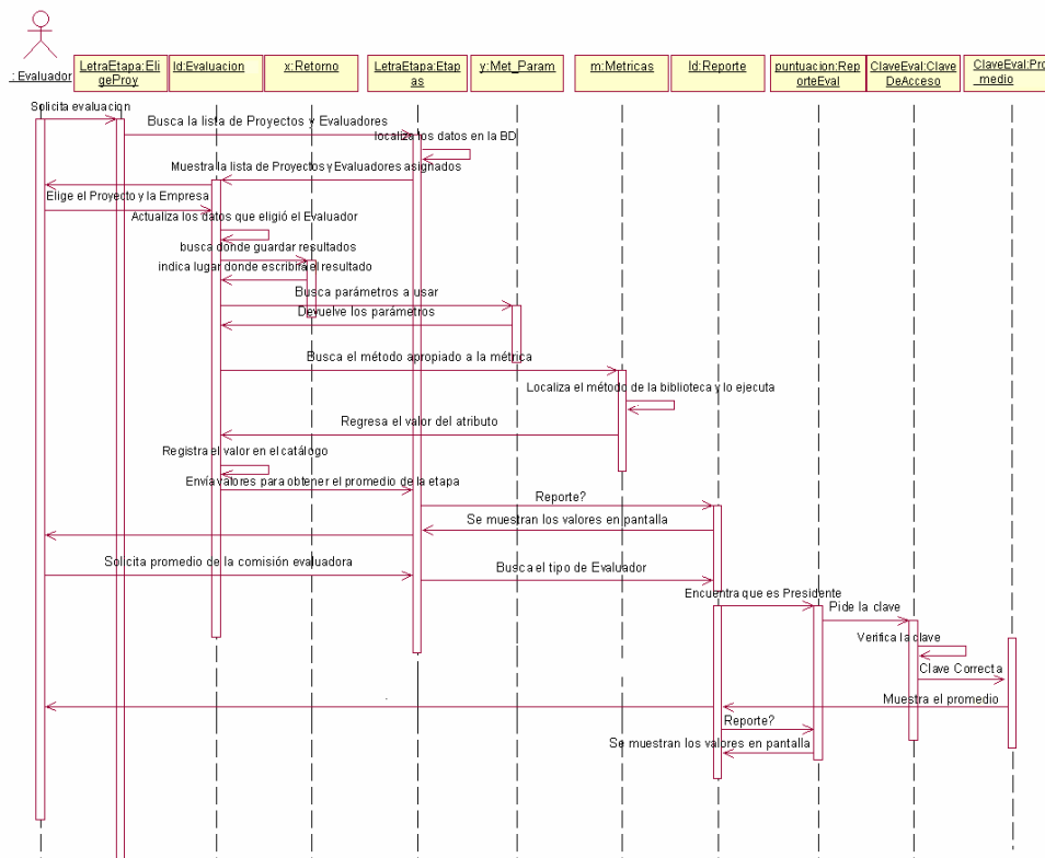
Figura 3.2 Diagrama de secuencia de la Evaluación individual.
