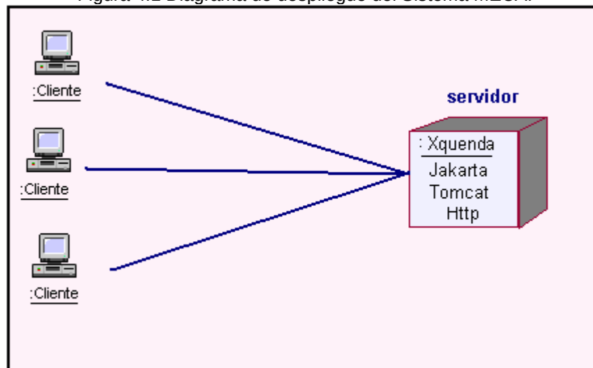
Figura 4.1 Diagrama de despliegue del Sistema MECA.
