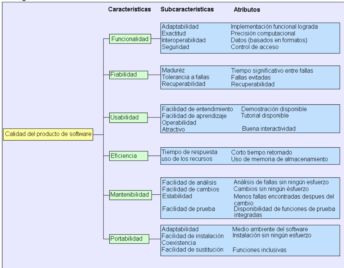
Figura 2.4 Modelo de Calidad de Software de la Norma ISO/IEC 9126.
