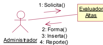
Figura AP.B.1 Diagrama de colaboración del Registro del Evaluador
