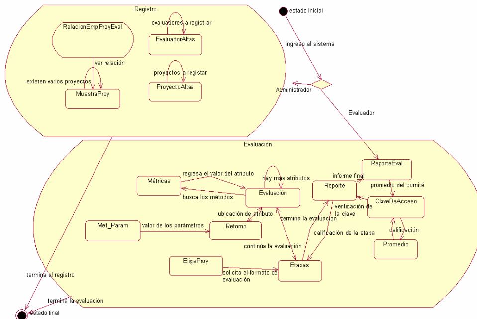
Figura 3.4 Diagrama de estados del Sistema MECA
