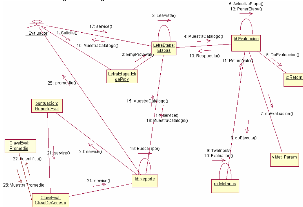
Figura 3.3 Diagrama de colaboración de la Evaluación
