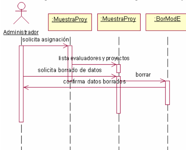
Figura AP.A.5 Diagrama de secuencia de la Asignación de Proyectos.
