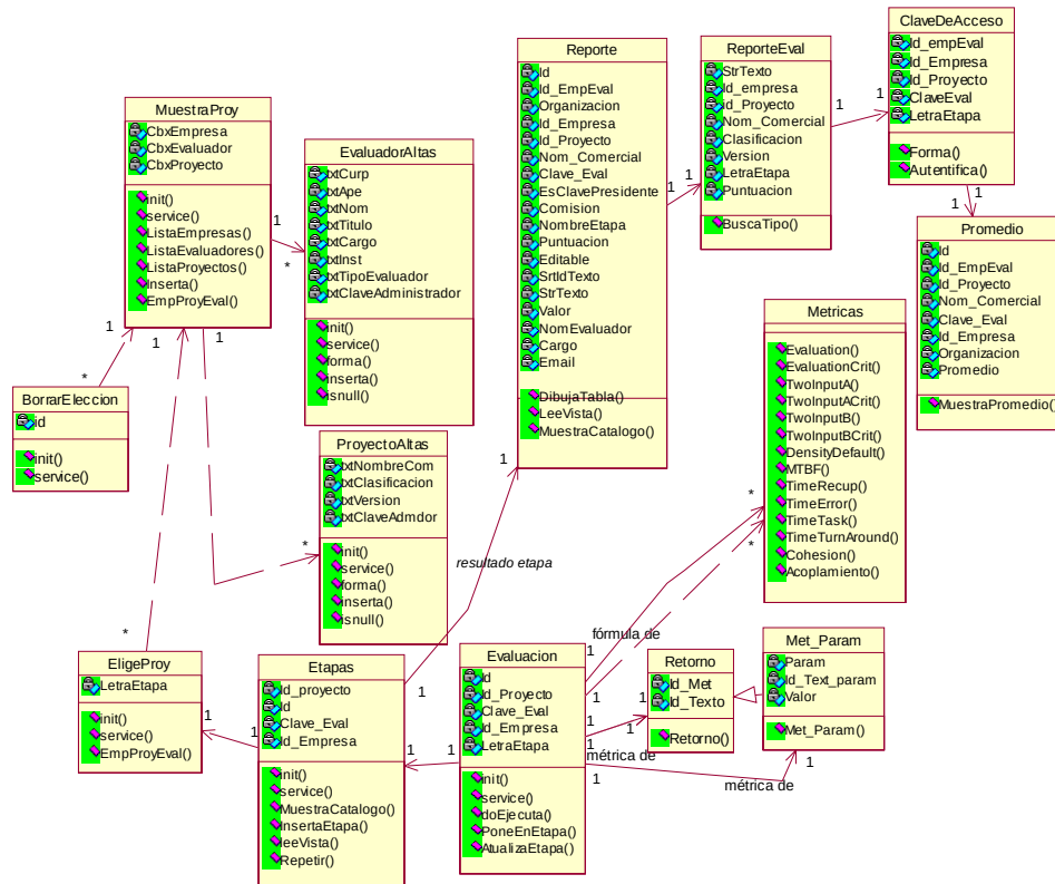
Figura 3.9 Diagrama de clases y relaciones del Sistema MECA.
