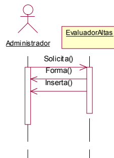
Figura AP.A.2 Diagrama de secuencia de bajo nivel de abstracción del Registro de Evaluadores.
