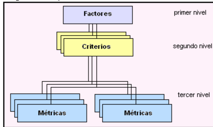
Figura 2.1 Esquema de la Calidad del Software de McCall
