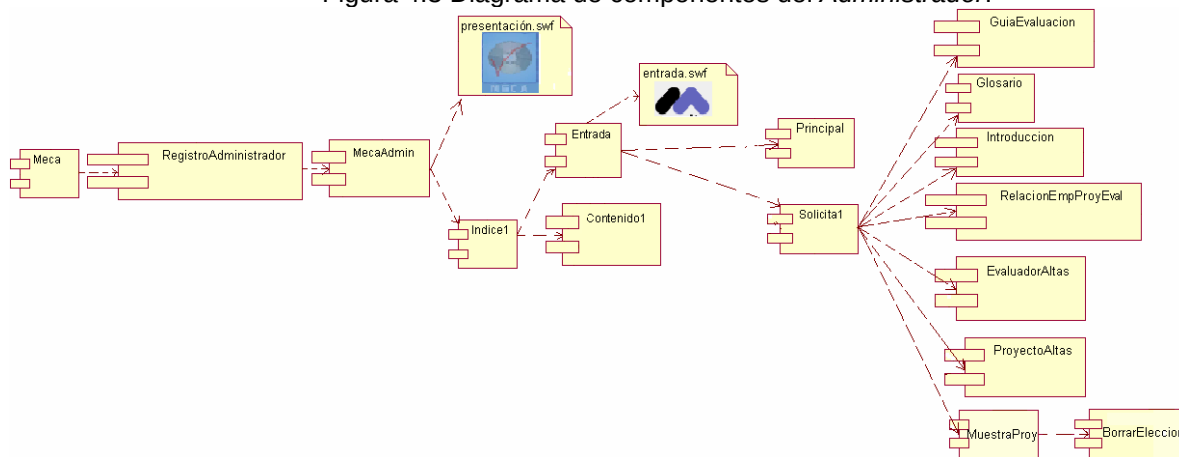
Figura 4.3 Diagrama de componentes del Administrador .
