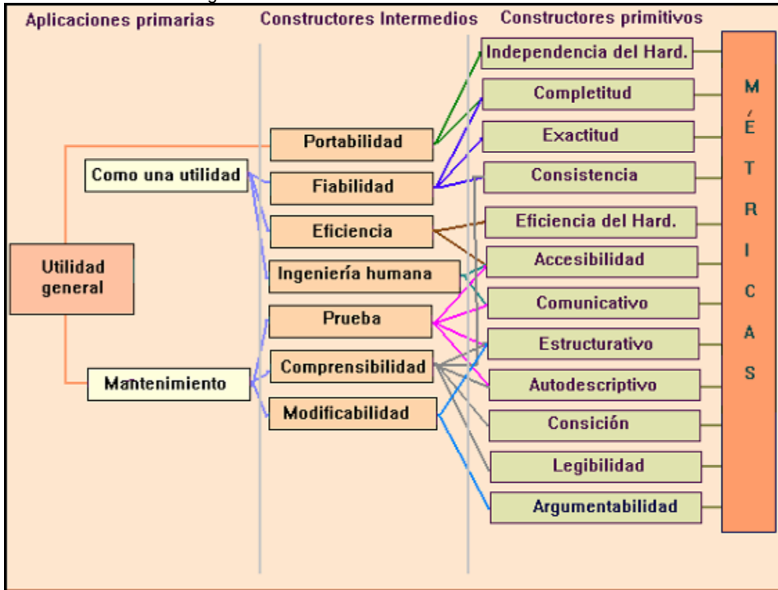
Figura 2.2 Modelo de Calidad de Software de Boehm
