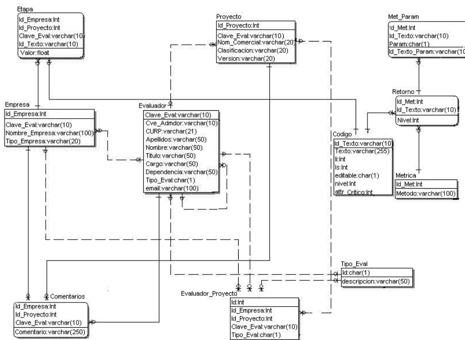
Figura 3.18 Modelo Lógico Entidad-Relación
