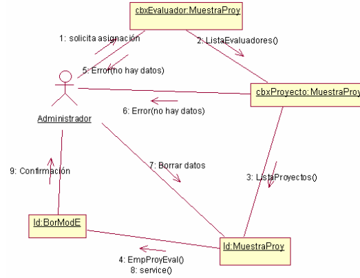
Figura AP.B.3 Diagrama de colaboración de la Asignación de Proyectos
