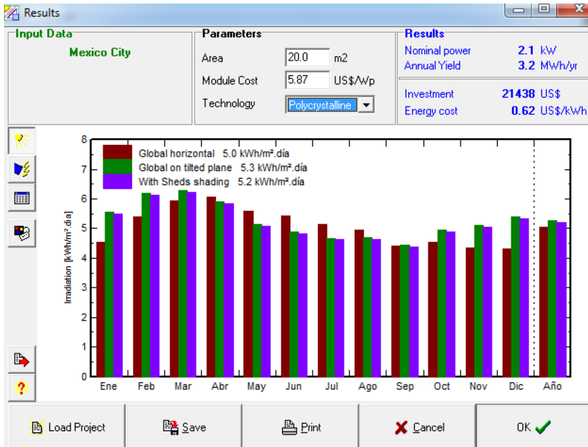
Fig. 69 Resultados Finales del pre dimensionamiento.
