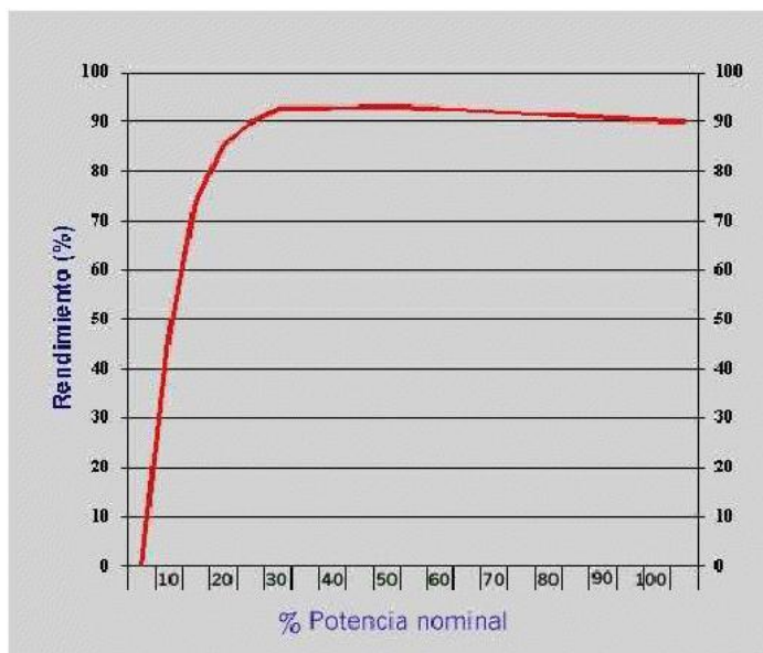
Fig. 45 Curva de rendimiento de un inversor.
