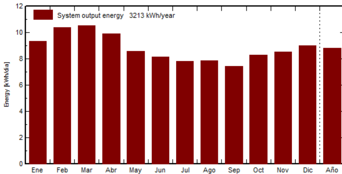
Fig. 70 Salida de energía eléctrica del pre dimensionamiento por mes en kWh/día.
