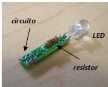
Fig. 84 LED, con resistor y circuito incluido. Fuente: FGRT11
