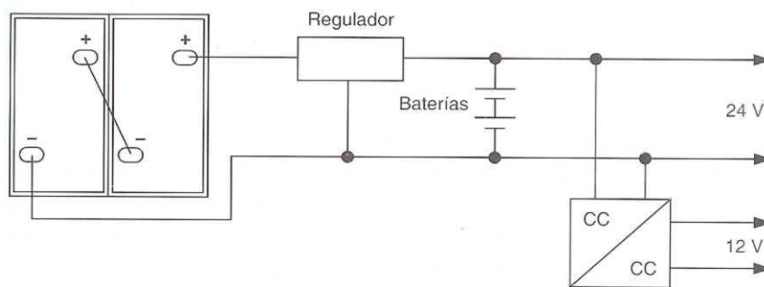
Fig. 44 Esquema de instalación fotovoltaica aislada con convertidor cc/cc.
