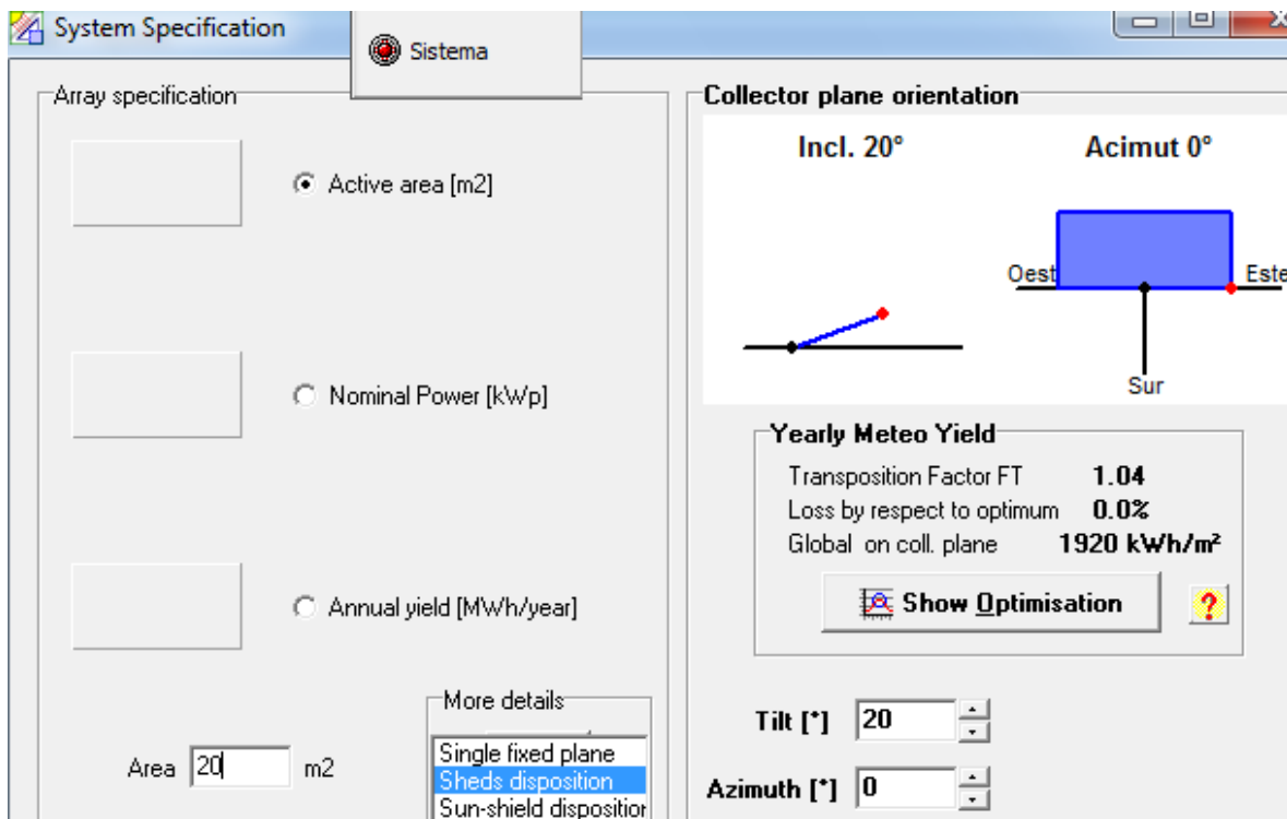
Fig. 64 Especificaciones del sistema (inclinación, orientación, área activa).
