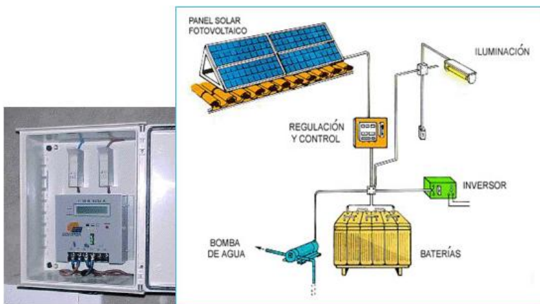
Fig. 43 Regulador/Ubicación del regulador en el esquema de conexión de una instalación fotovoltaica aislada.
